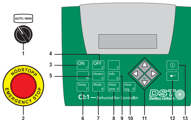
ABB. 13: SPS-Tasten
