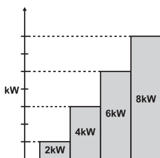
ABB. 29: Binärregelung
