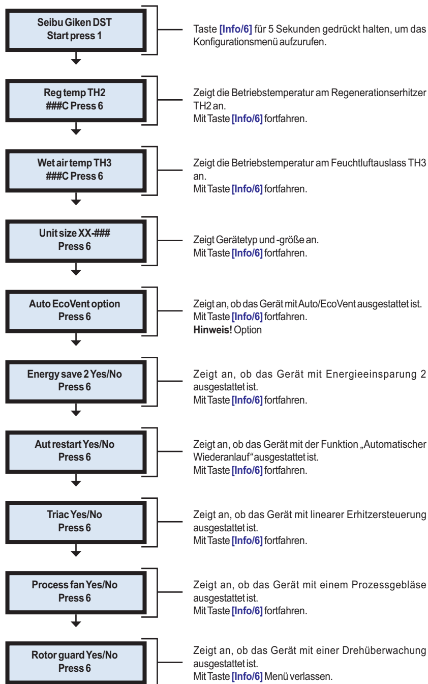
ABB. 23: Geräteeinstellungen überprüfen
