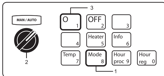
ABB. 14: Entfeuchter in Betriebsart AUTO/OFF oder AUTO/VENT starten
