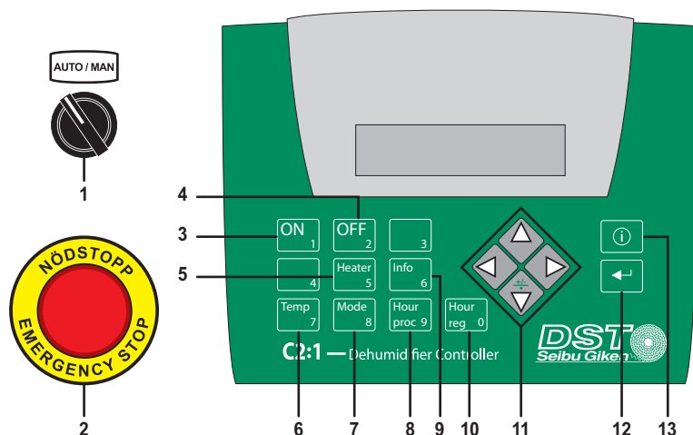
ABB. 13: SPS-Tasten
