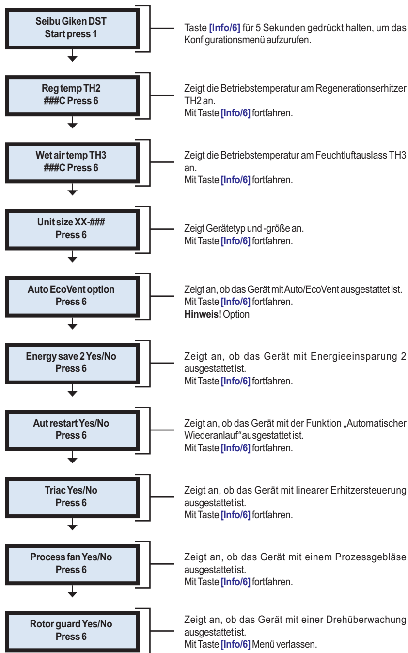
ABB. 23: Geräteeinstellungen überprüfen
