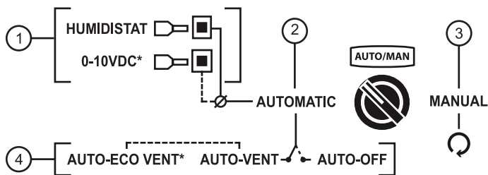
ABB. 24: Übersicht der automatischen und manuellen Funktionen
