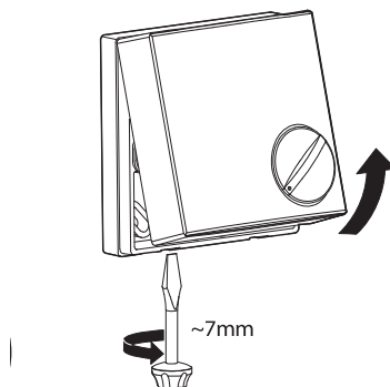
ABB.16: Abdeckung
