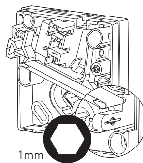
FIGUR 17: Kalibreringsskruv
