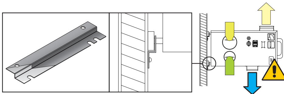
IMAGE 11: Support pour montage mural
