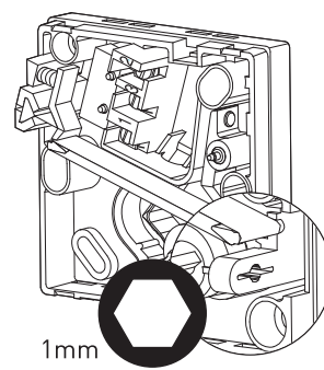
FIGURA 17: Tornillo de calibración
