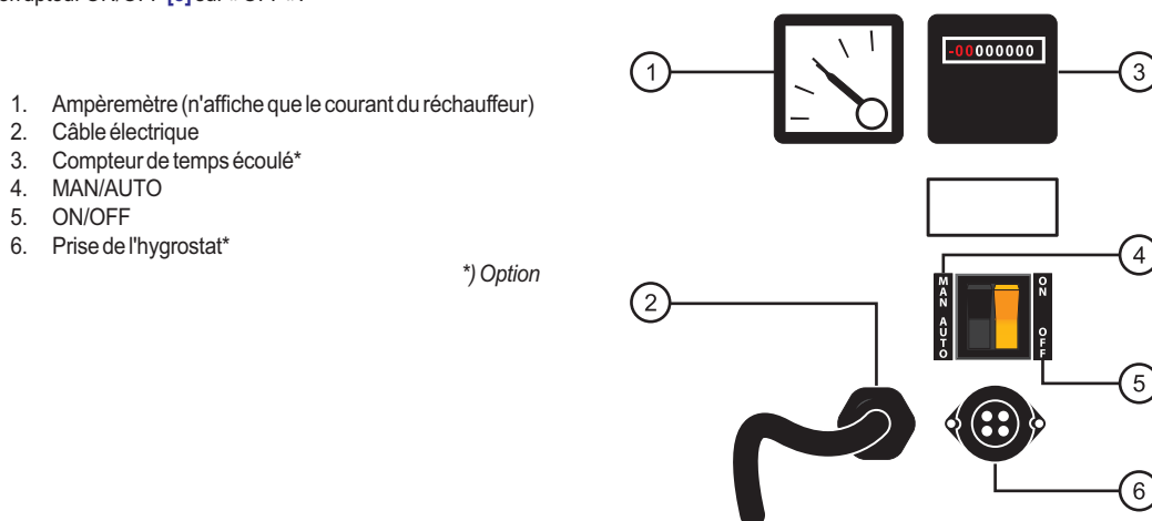
IMAGE 9: Panneau de commande
