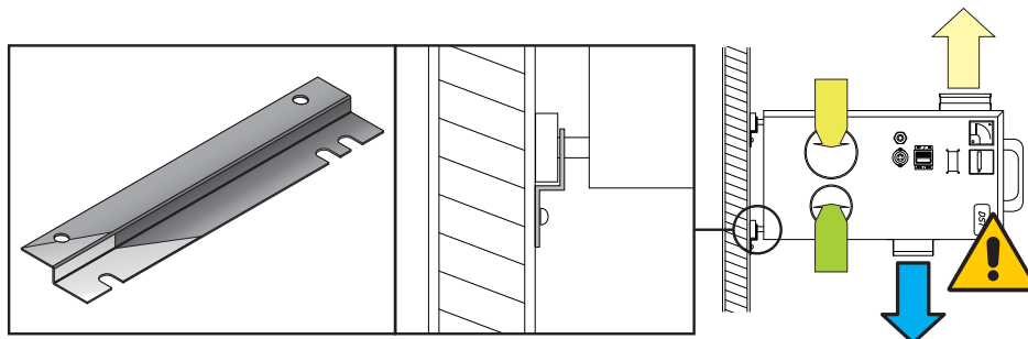
FIGUR 11: Stålfästen för väggmontering
