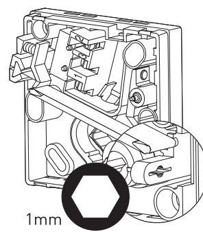
FIGUR 15: Kalibreringsskruv
