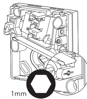
ABB.15: Kalibrierschraube
