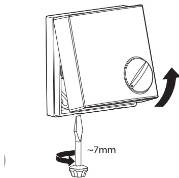
ABB. 14: Abdeckung
