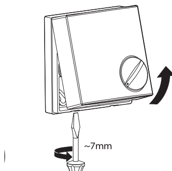
FIGURA 14: Tapa
