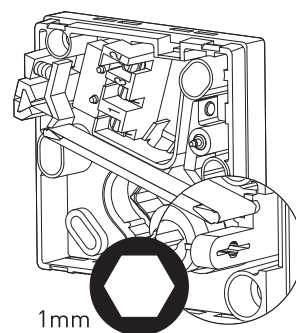
FIGURA 15: Tornillo de calibración
