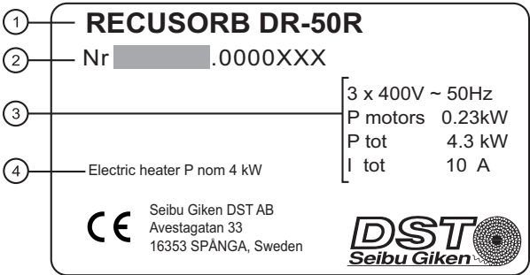
ABB. 1: Typenschild
