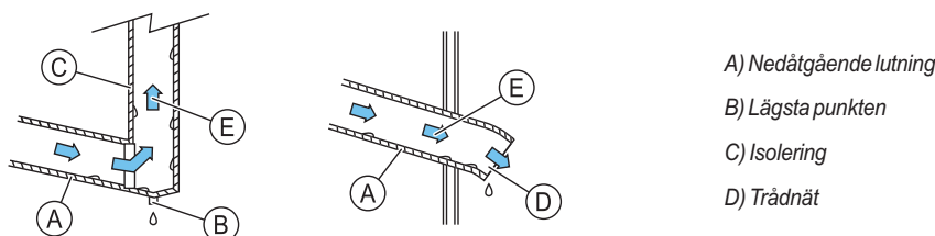
FIGUR 6: Installation med svag lutning och ledning uppåt
