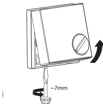
FIGURA 15: Tapa
