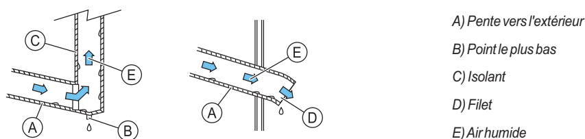
IMAGE 6: Installation de la gaine de sortie d'air humide
