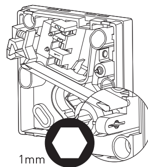
ABB. 16: Kalibrierschraube
