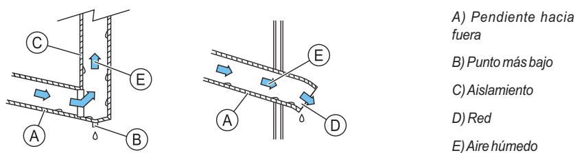
FIGURA 6: Instalación de conducto de salida de aire húmedo
