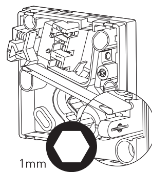
FIGUR 16: Kalibreringsskruv
